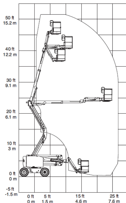
Z-45/25J 動作範圍圖
